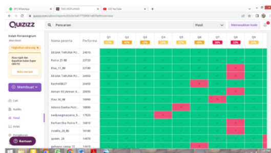
Gambar 3 Analisis Butir Soal
